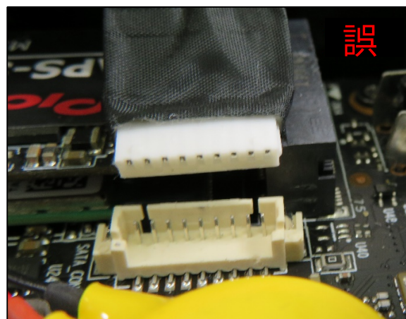
14. 上の写真は誤った挿入方法です。コネクタが上下逆になっています。
