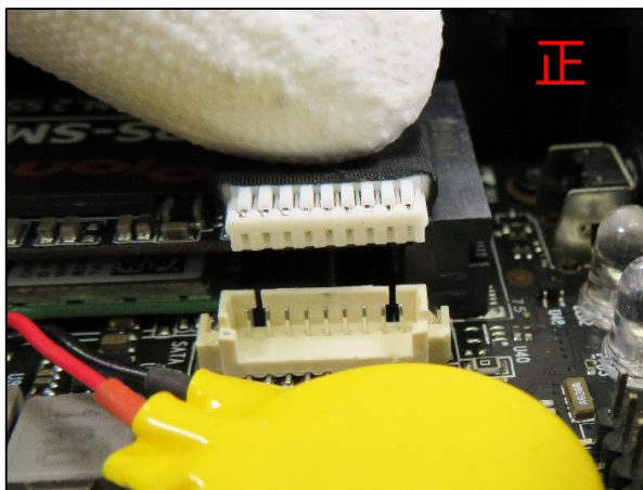
13. マザーボードの 9PIN インターフェイスに HDD ケーブルを挿入します。写真の様にコネクタの上下の向きにご注意ください。
